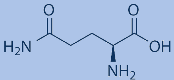
L-glutamine
